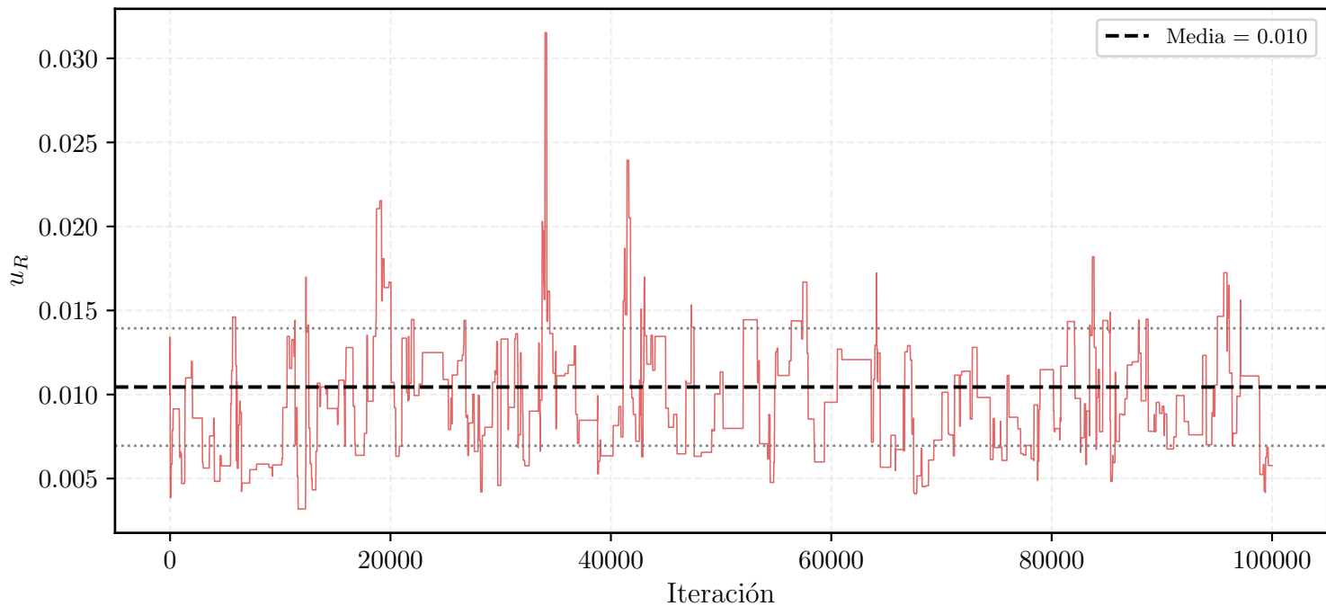
Cadena MCMC - u_R
